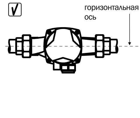
Рис.4 Установка циркуляционного насоса.
