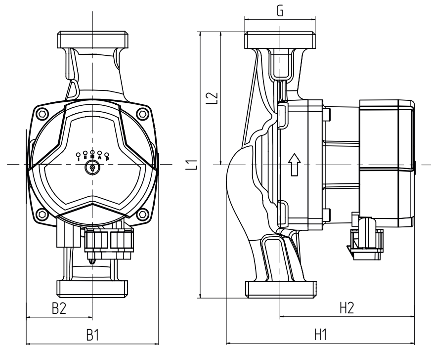
Рис.1 Обозначение монтажных размеров насоса.
