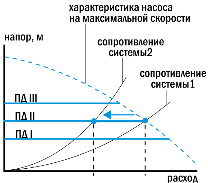
Рис.10 График работы насоса в режиме ПД.
