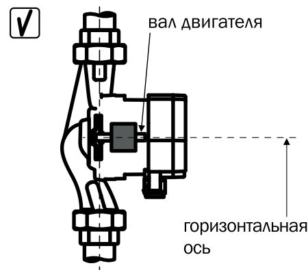
Рис.4 Установка циркуляционного насоса.
