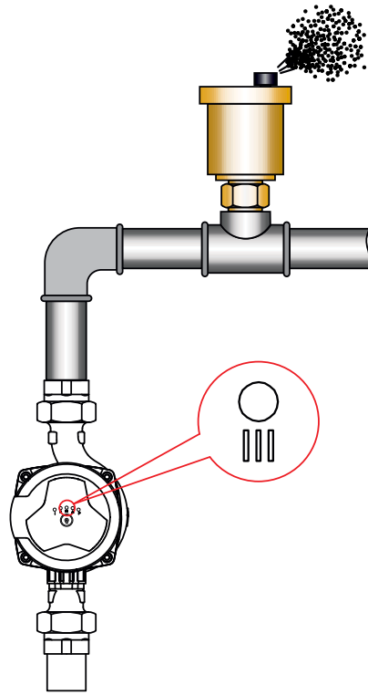
Рис.2 Удаление воздуха из корпуса насоса.
