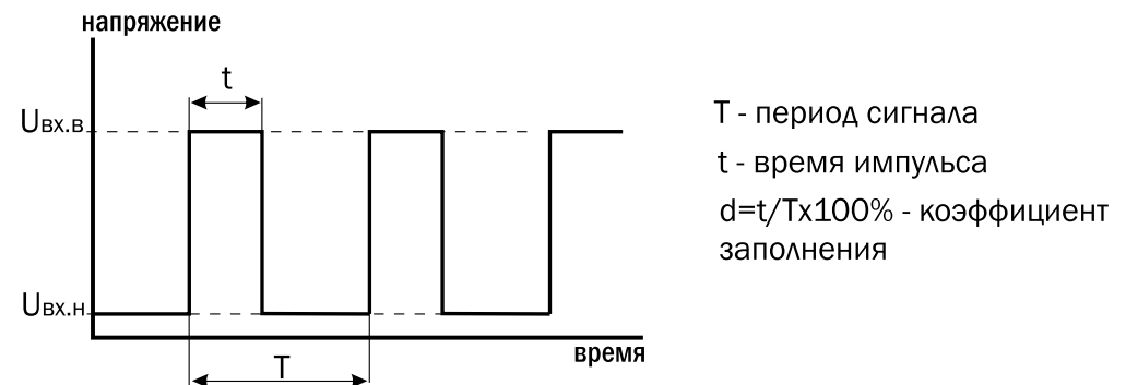
Рис.13 Характеристики ШИМ-сигнала.
