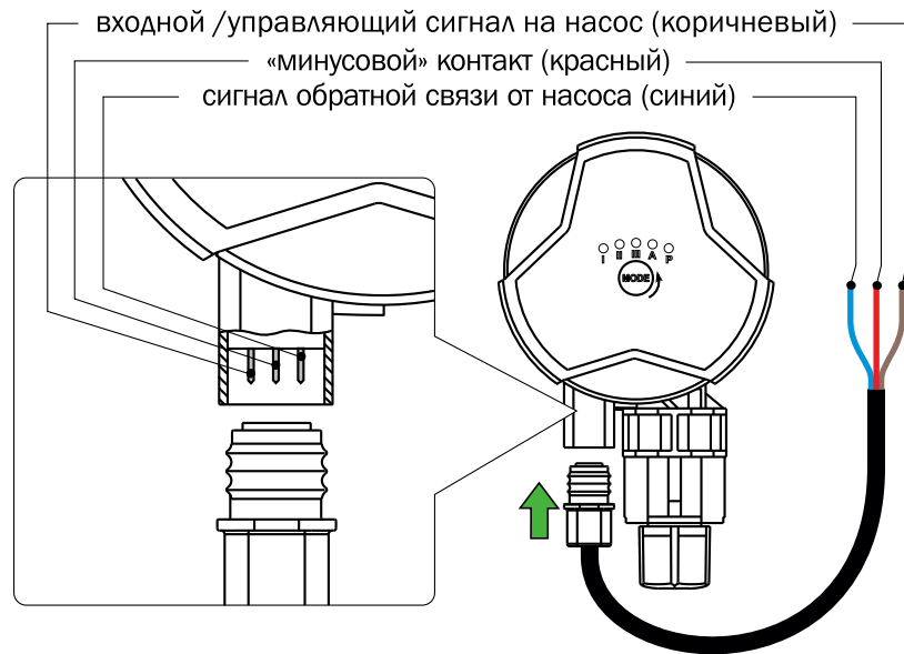
Рис.8 Схема подключения ШИМ-сигнала.
