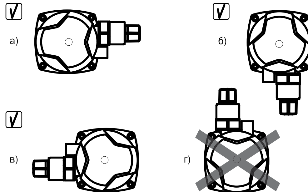
Рис.5 Правильное расположение насоса.
