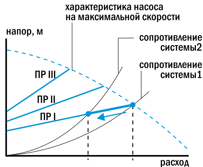
Рис.11 График работы насоса в режиме ПР.
