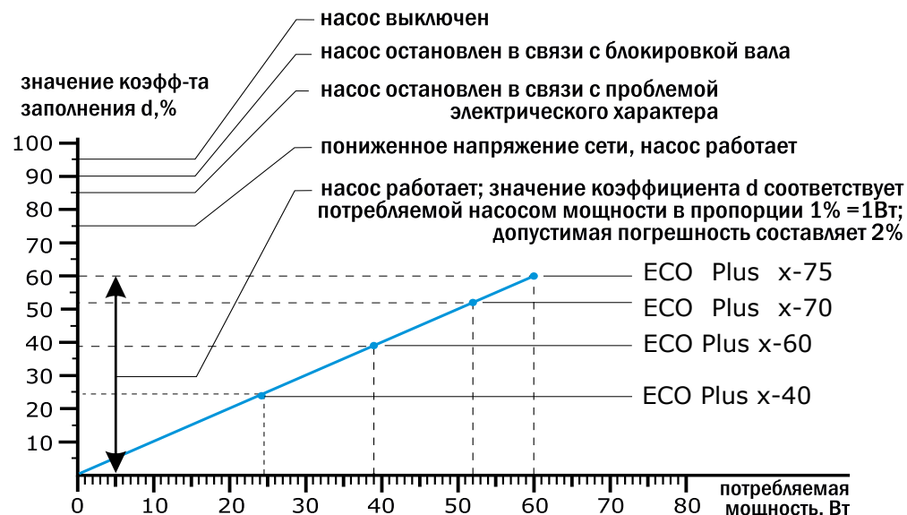
Рис.15 Зависимость коэффициента заполнения от состояния насоса.
