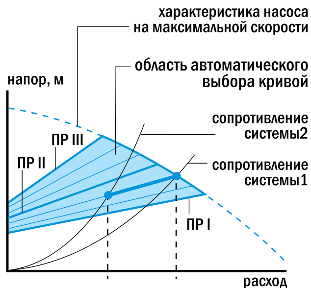
Рис.12 График работы насоса в режиме АВТО.
