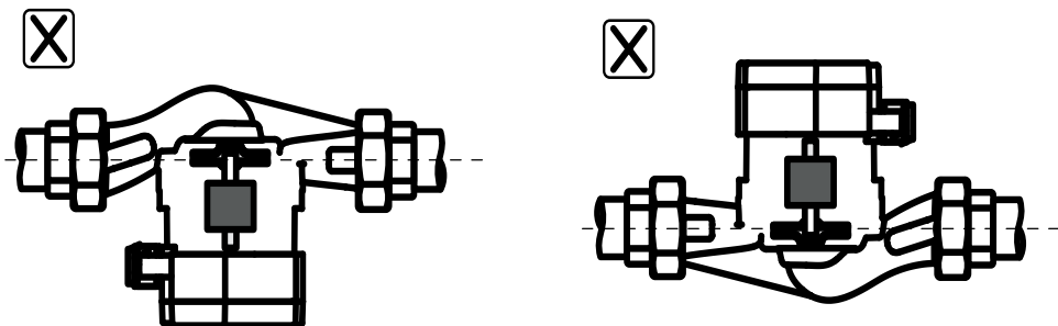
Рис.4.1 Неправильная установка насоса.
