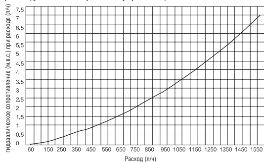
Кривая гидравлического сопротивления устройства в целом
