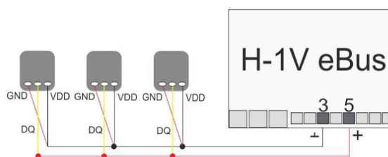
Датчик DS18B20
