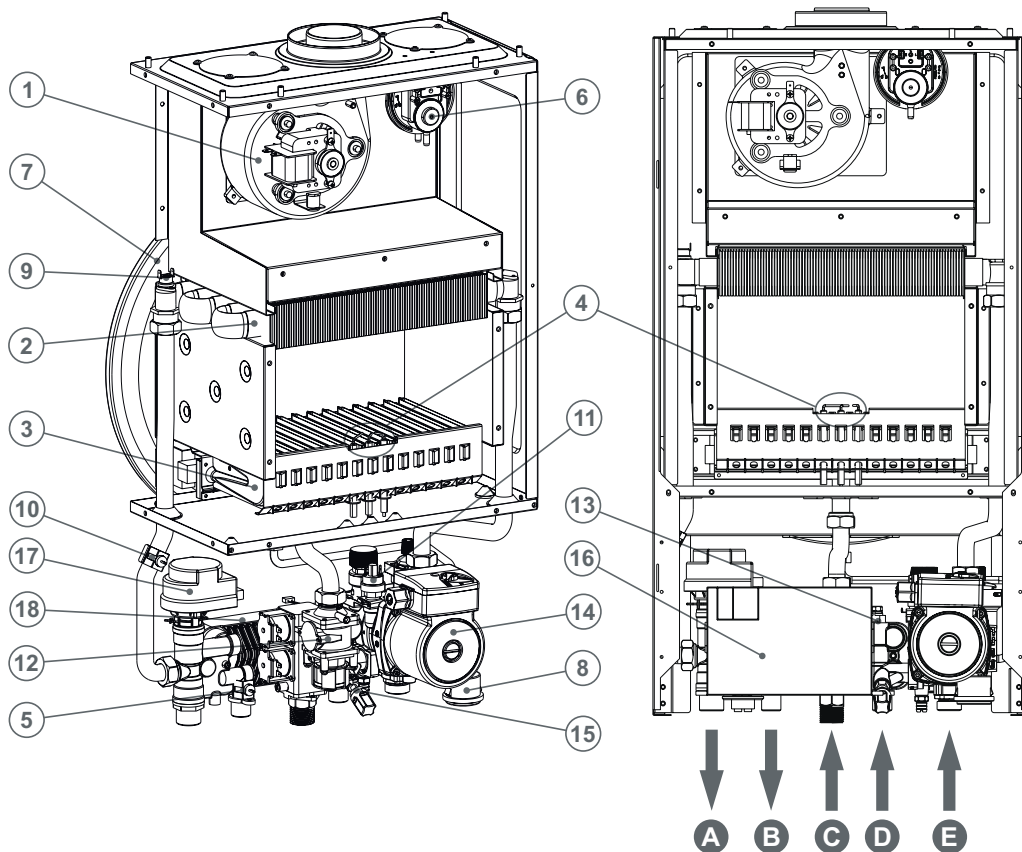
Рисунок 4.2. Общий вид котла ОЧАГ-28Е
