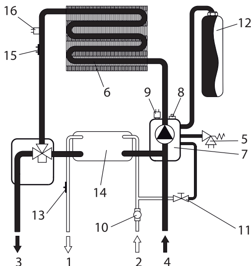
Гидравлическая схема в режиме отопления
