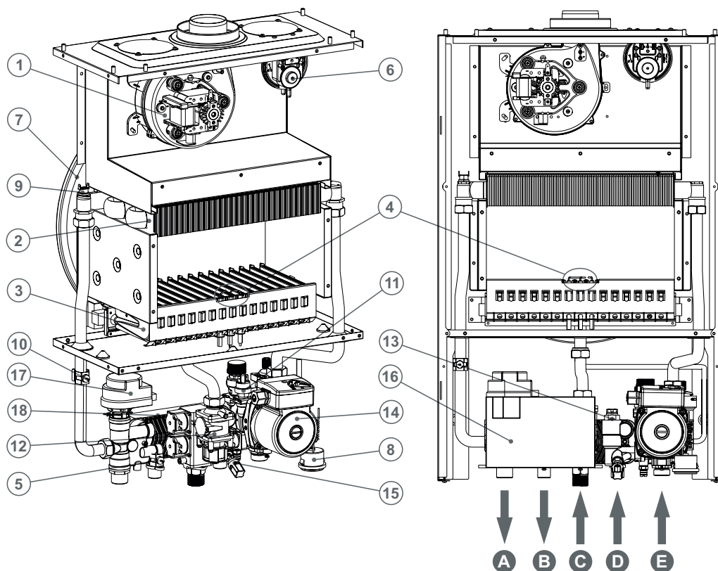
Рисунок 4.3. Общий вид котла ОЧАГ-32Е
