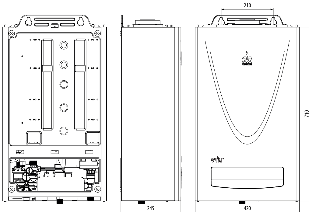
Рисунок 1.1. Габаритные и присоединительные размеры котлов ОЧАГ-10Е/13Е/16Е/20Е/24Е
