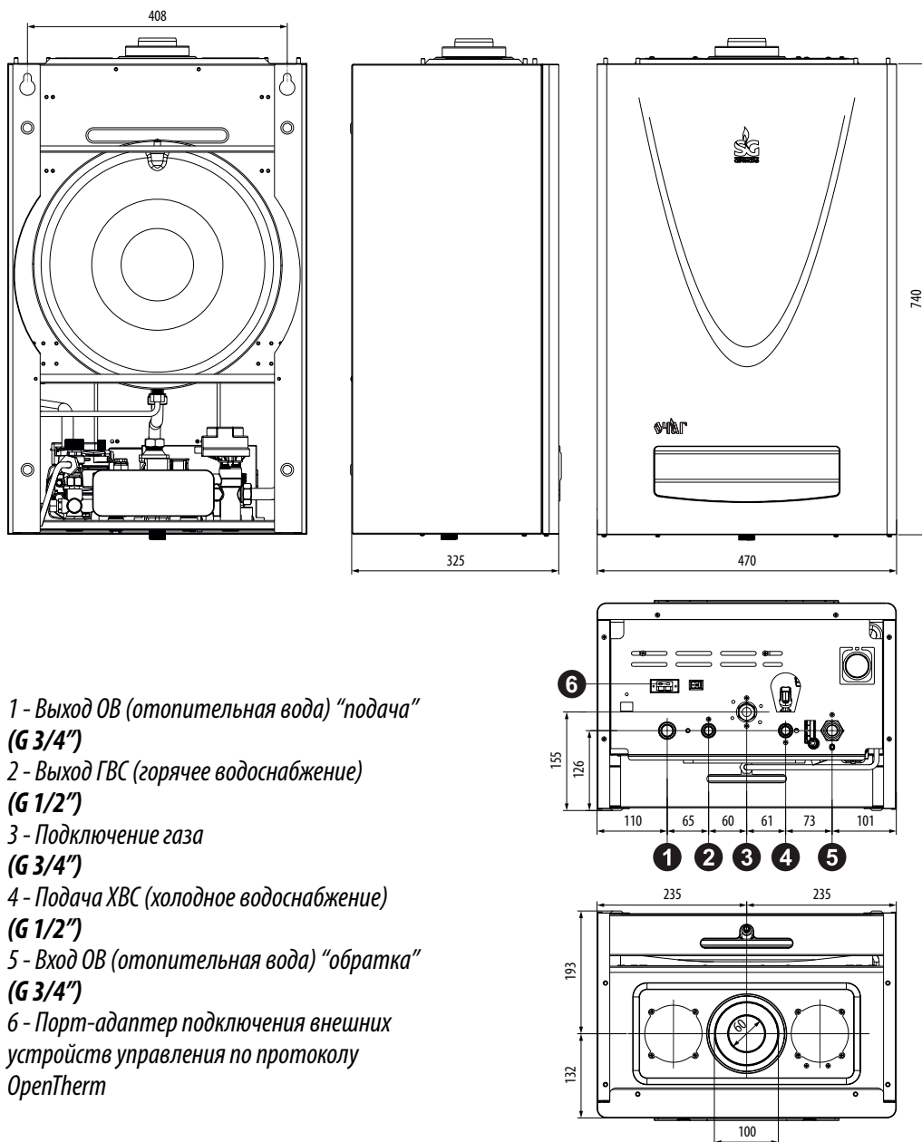
Рисунок 1.3. Габаритные и присоединительные размеры котла ОЧАГ-32Е
