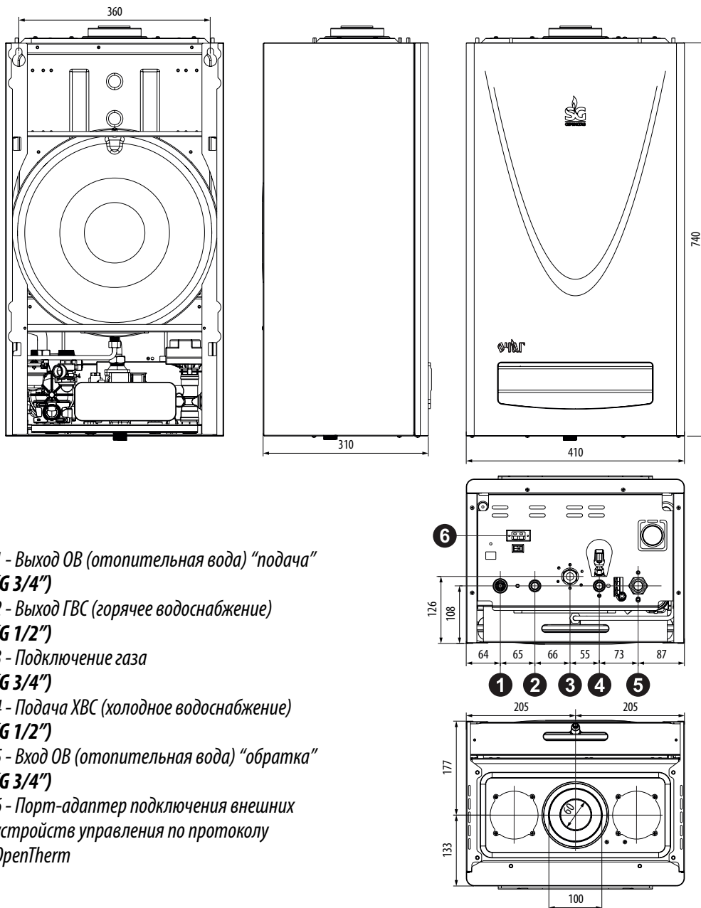
Рисунок 1.2. Габаритные и присоединительные размеры котла ОЧАГ-28Е
