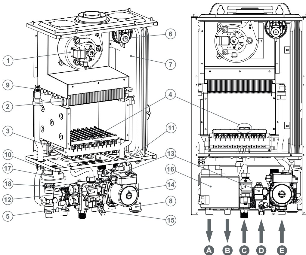
Рисунок 4.1. Общий вид котлов ОЧАГ-10Е/13Е/16Е/20Е/24Е
