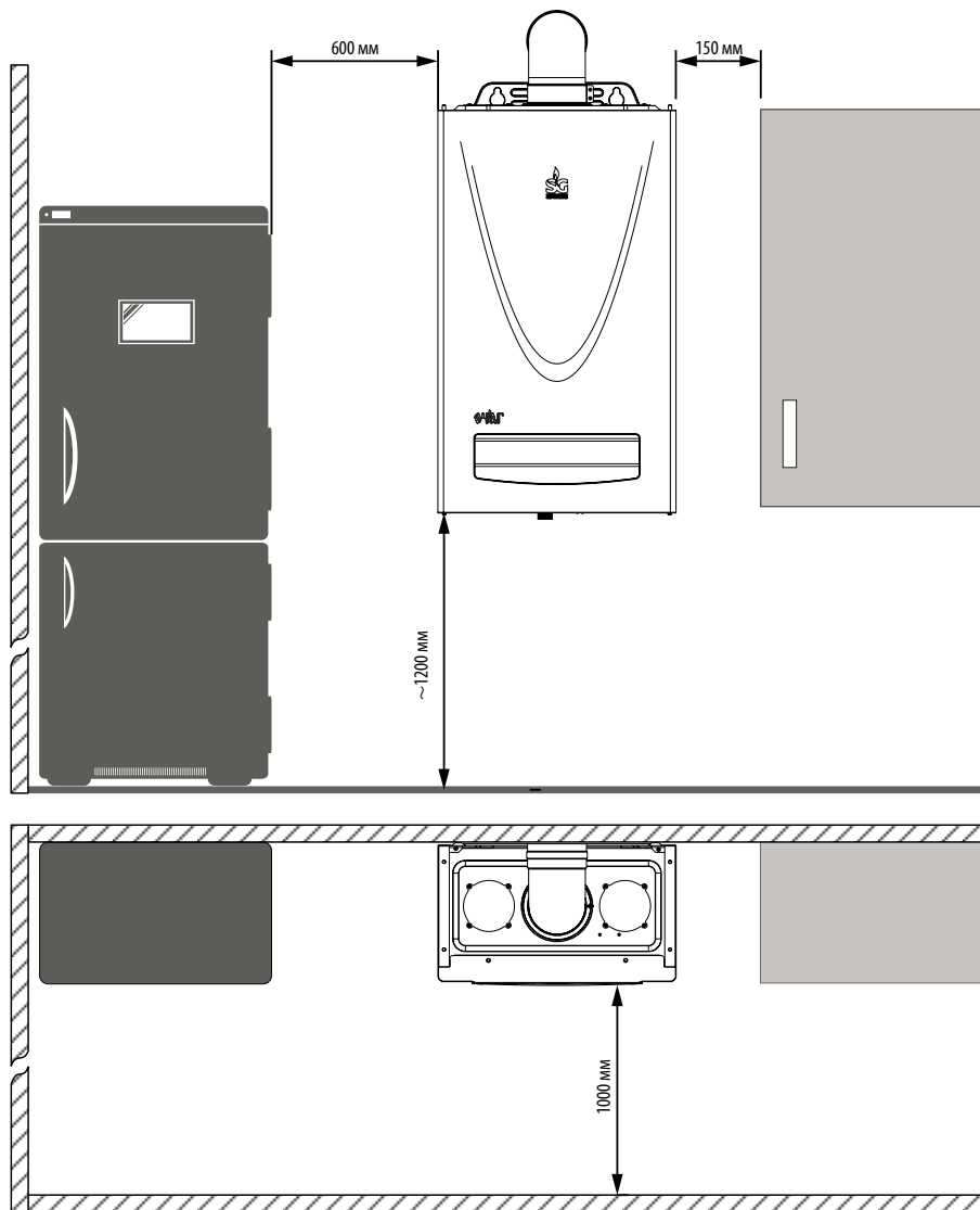
Рисунок 6. Размещение котла
