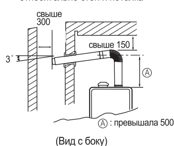
Расположение дымохода относительно стен и потолка
