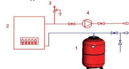
Схема подключения бака Рис.2
