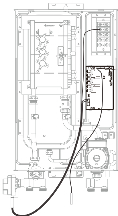
Рис. 17. Подключение датчика бойлера
