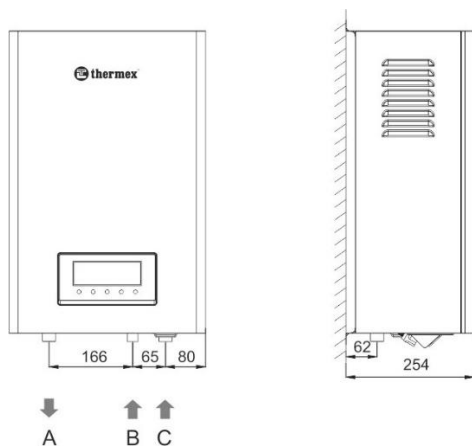
Рис. 7. Присоединительные размеры
