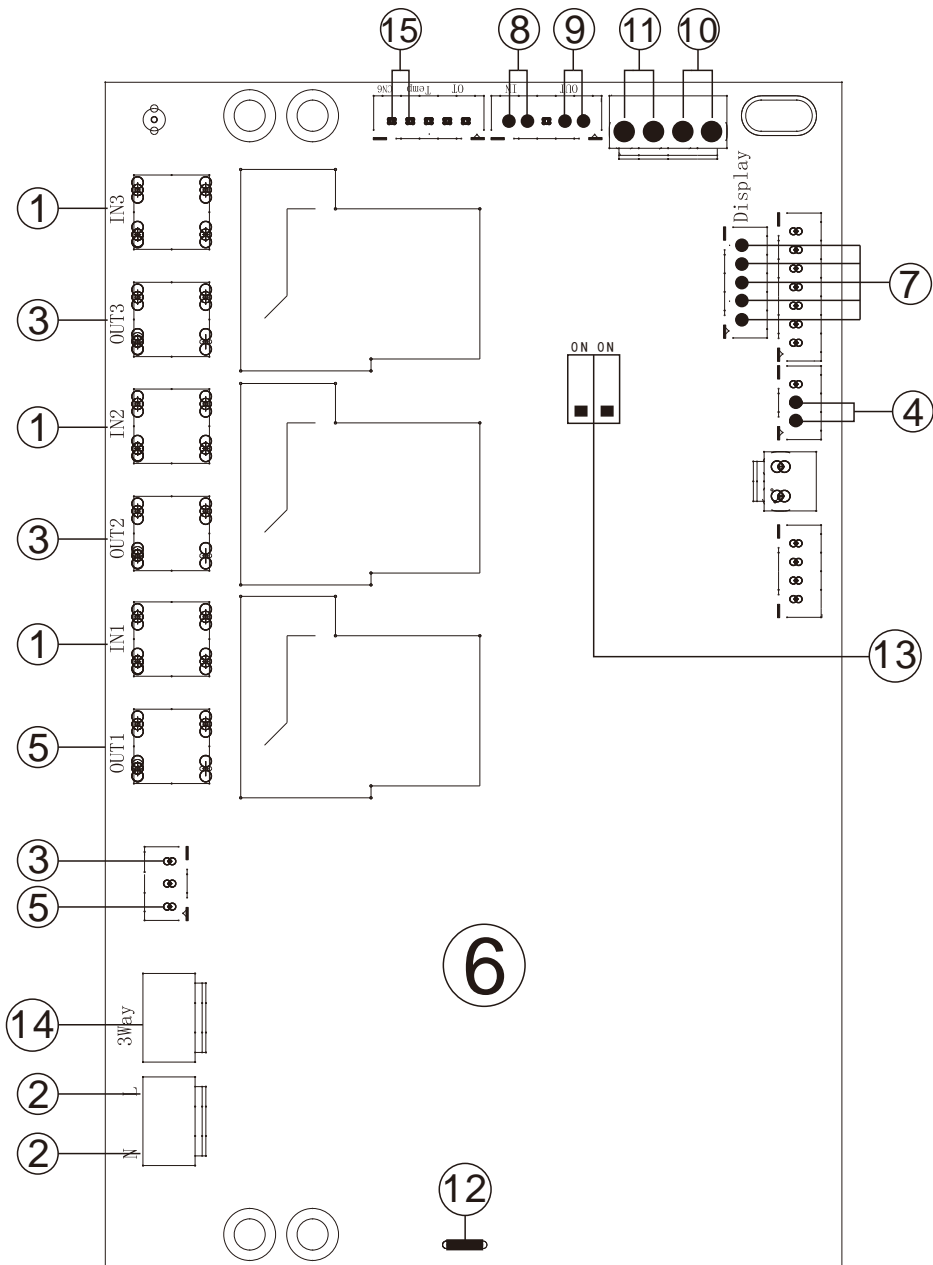
Рис. 20. Электрическая схема основной платы управления
