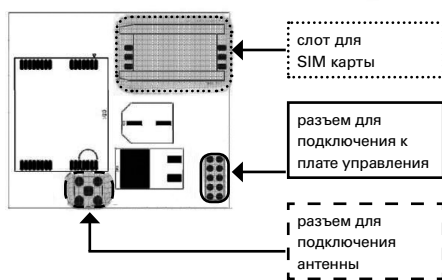
Рис. 1. Вид платы GSM-модуля
