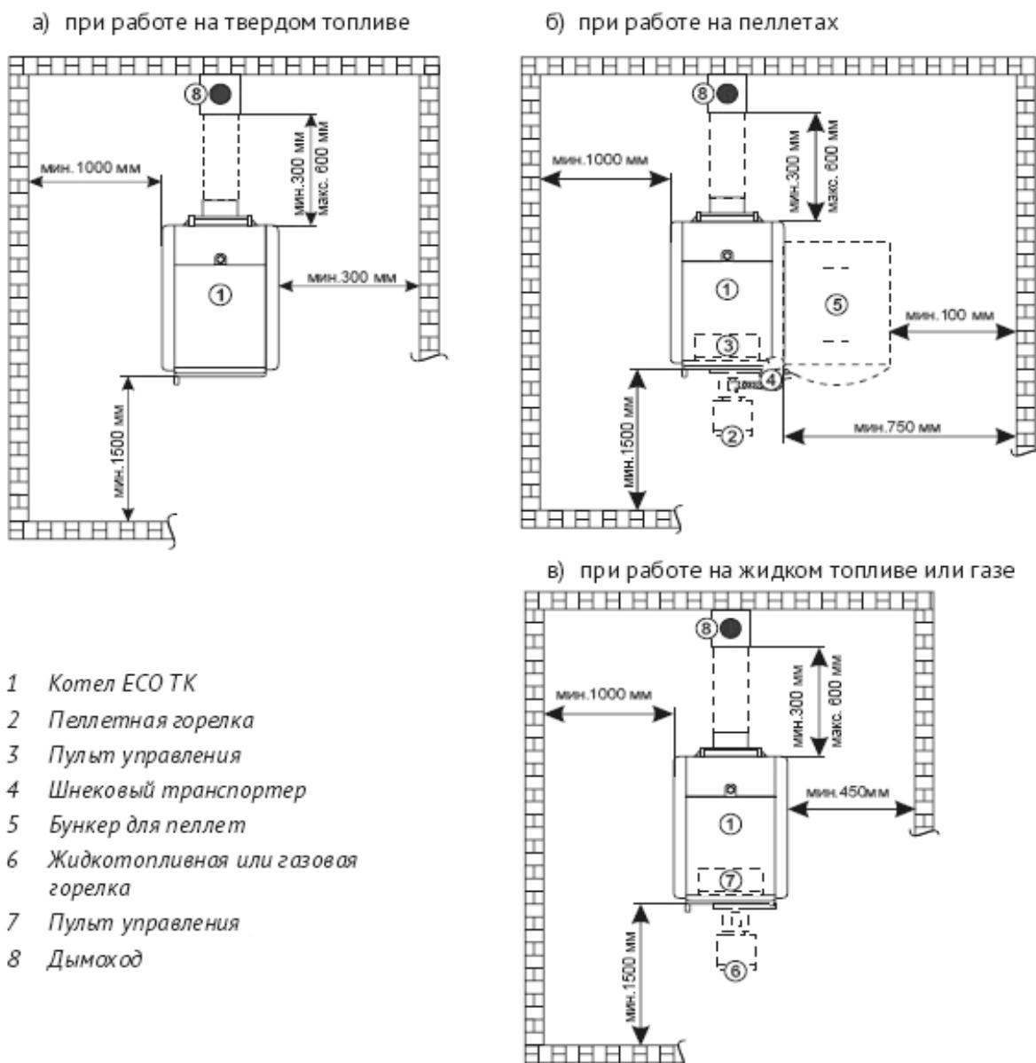
Рисунок 2. Минимальные расстояния от котла до стен котельной
